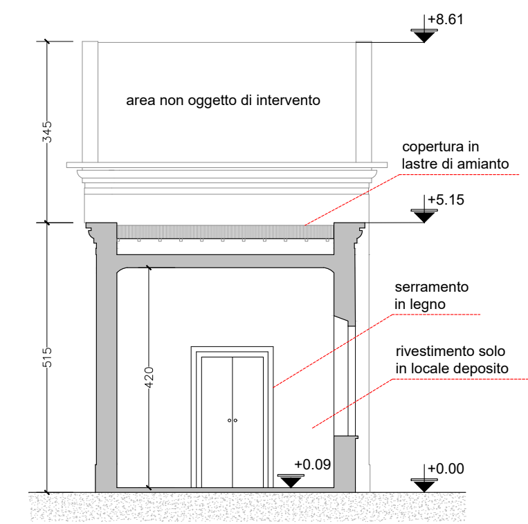
SEZIONE BB
