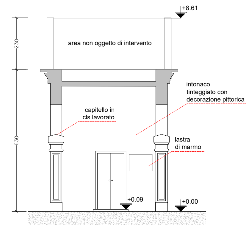
SEZIONE AA
